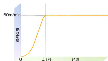
FJV-200 UHS 送り速度特性
