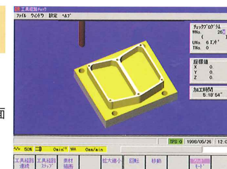
ツールパスソリッドチェック画面
