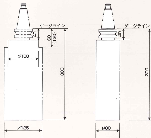
隣接ポケットツール無し
